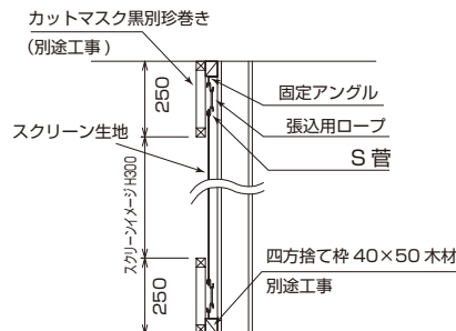
■ 断面詳細図
