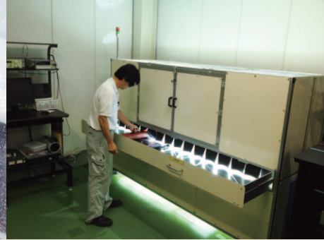
モバイルソーラー発電試験
