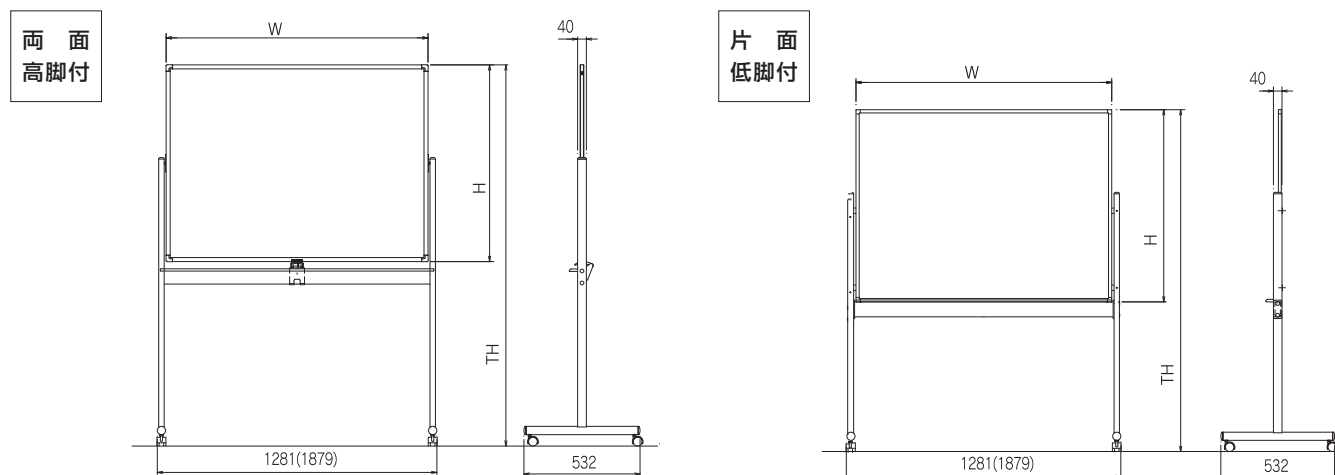
カラーボード「いろいろ」外形寸法図
