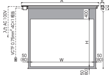
■外形寸法図
