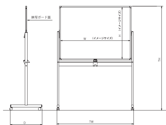
スクリーンボード「まくいた」外形寸法図
