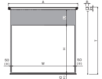
■外形寸法図
