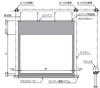
■外形寸法図
