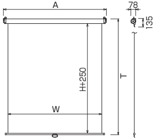
■外形寸法図
