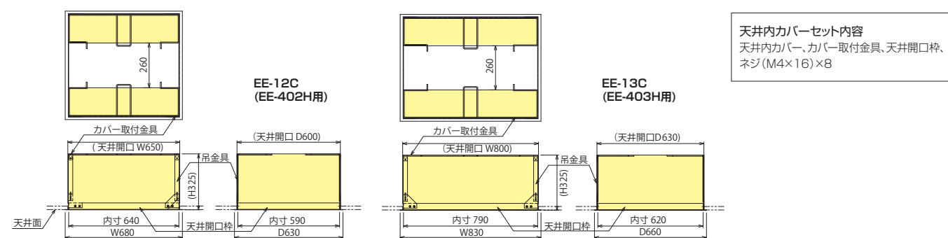
天井内カバー (オプション) 外形寸法図 天井内カバー / 黄色部
