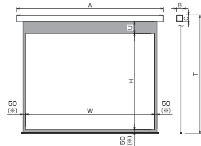
■外形寸法図
