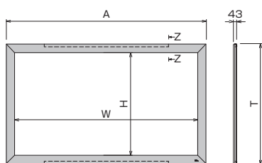
■ 外形寸法図
