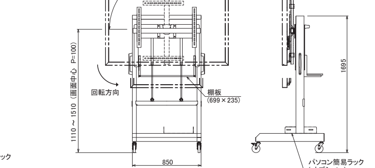
DSE-Kシリーズ (ディスプレイ回転型)
