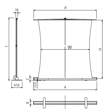
■外形寸法図
