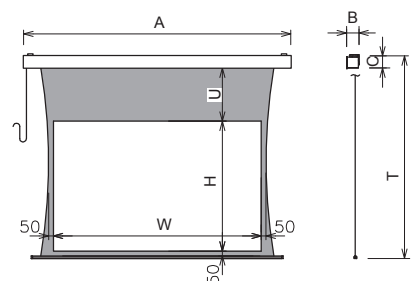
■外形寸法図
