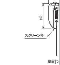
■Z-Z断面図
