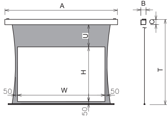
■外形寸法図
