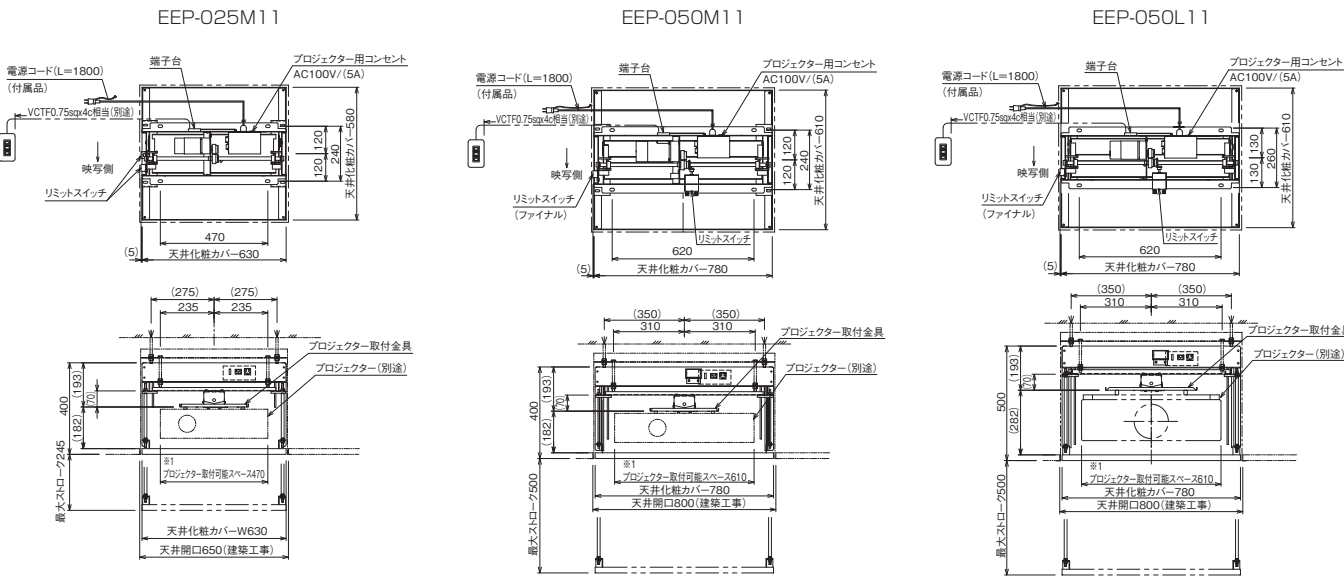
外形寸法図
