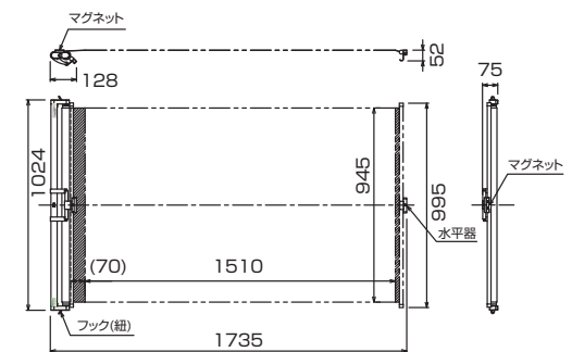
■外形寸法図
