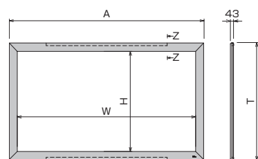
■外形寸法図
