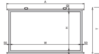
■外形寸法図
