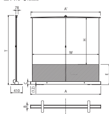
■外形寸法図
