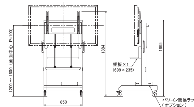
DSE-Fシリーズ (ディスプレイ固定型)
