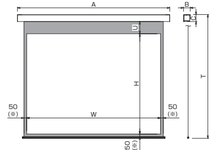
■外形寸法図
