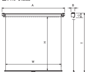
■外形寸法図
