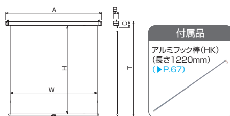
■外形寸法図
