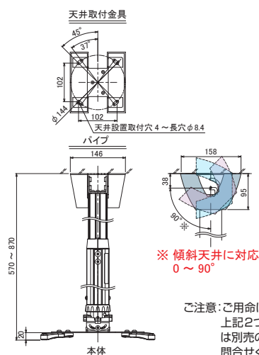
パイプセット外形寸法図 (PPC2555)
