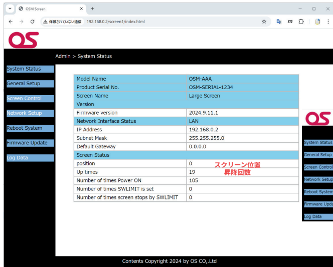
WEBブラウザ機能（System Status画面とスクリーン操作画面）
