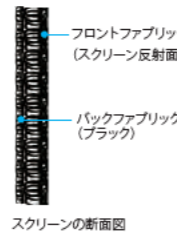
スクリーンの断面図
