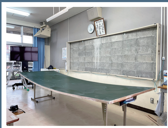
実際の施工風景 ※備品は学校側の許可を得て使用しています 作業完了後、清掃します
