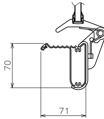
A-A 断面
