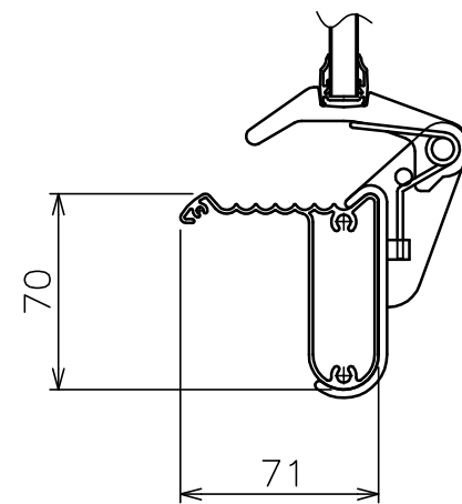
A-A 断面
