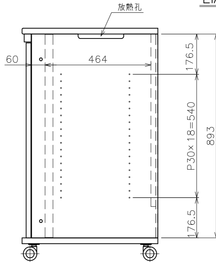
EIA 詳細図
