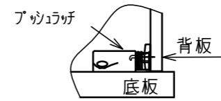
b部詳細
