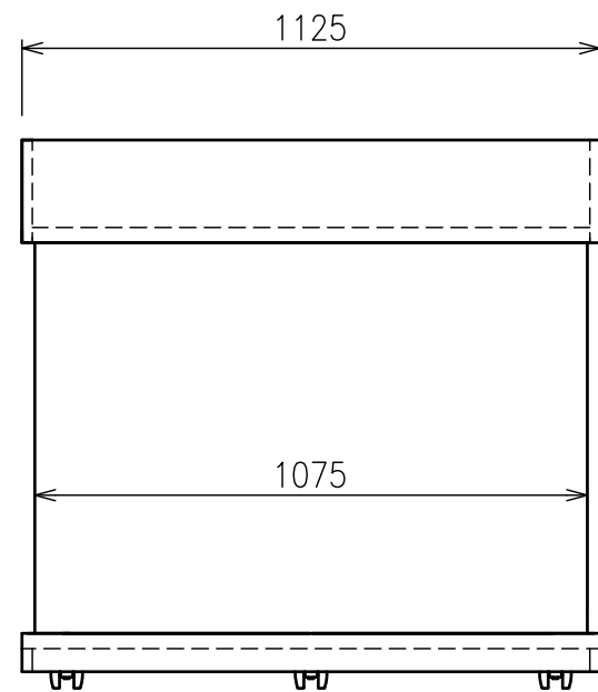
背面図
