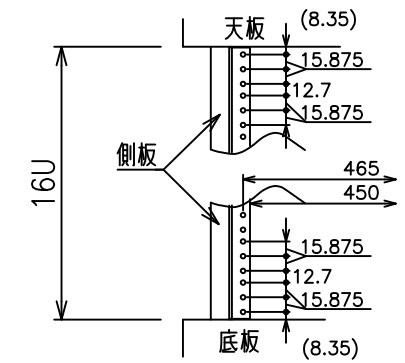
E I A金具 詳細図
