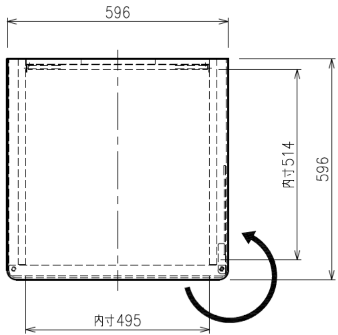
扉270度回転
