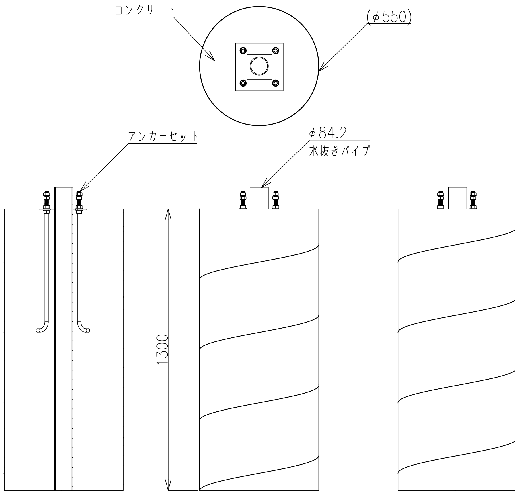
断面図
