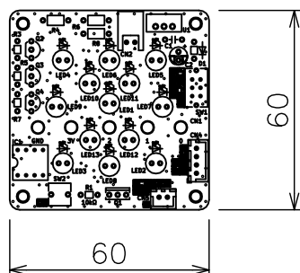
黒色 プリント基板 (t=1.6)×1
