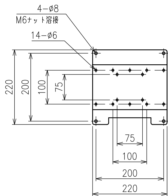
アタッチメントプレートA (DH-10A)
