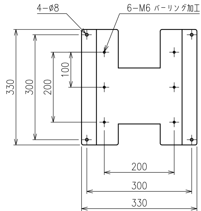
アタッチメントプレートB (DH-10B)
