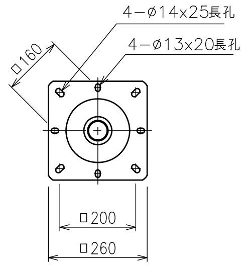
矢視 A - A
