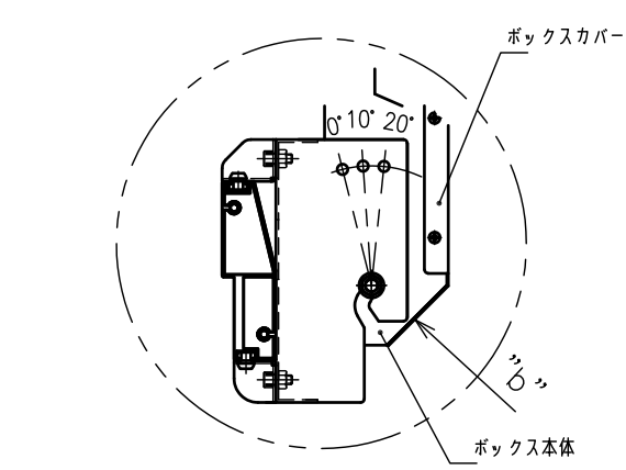
"a"詳細図 (取付金具とアルミフレームの連結)
