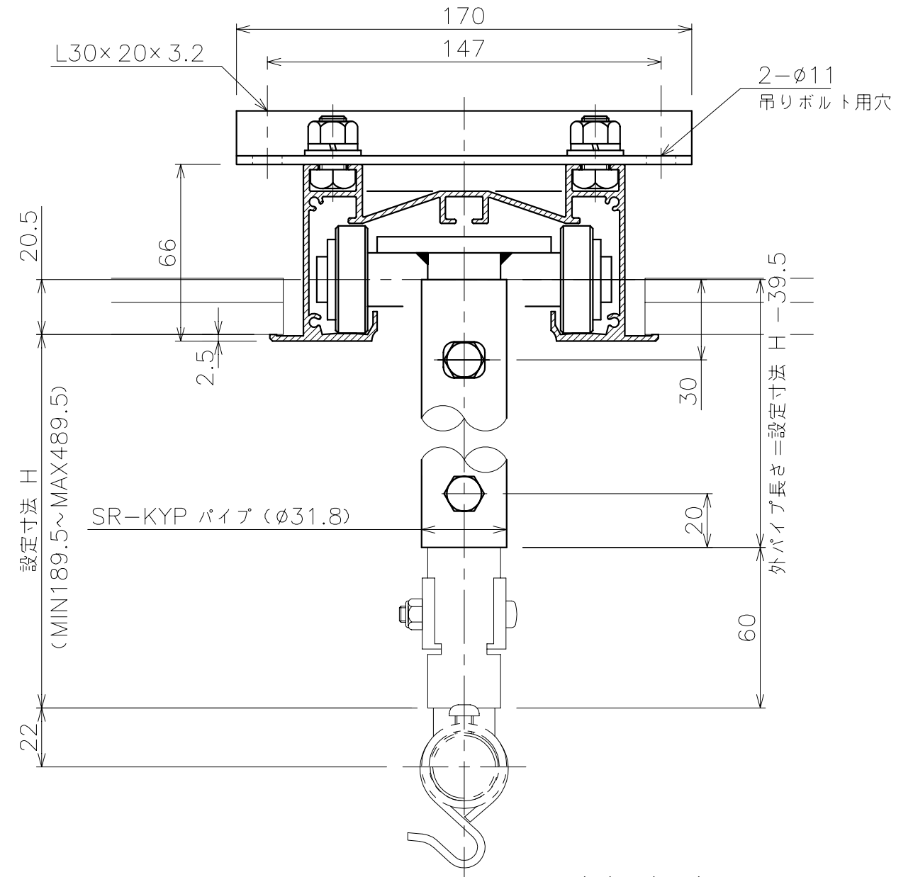
矢視 A-A
