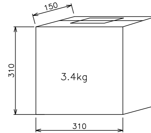
梱包仕様図(1/8)
