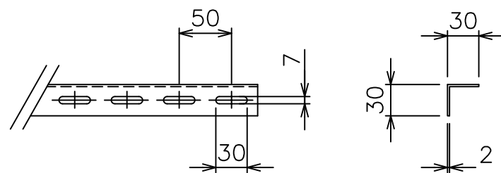
スクリーン取付金具詳細
