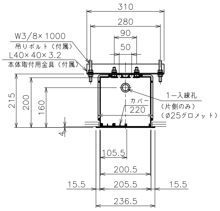
側面図詳細
