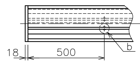
矢視 B
