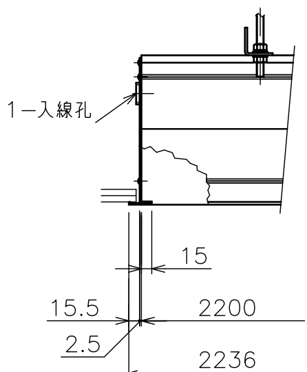
”a”部詳細
