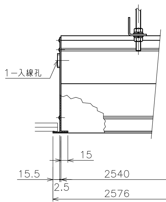
”a”部詳細
