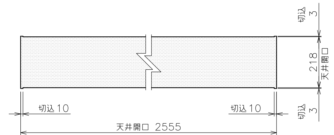
天井開口 KEYPLAN
