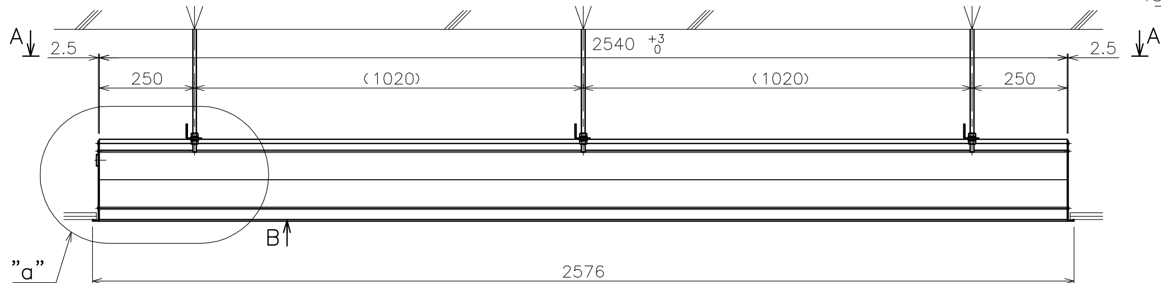
矢視 A - A
