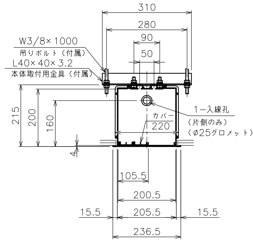
側面図詳細
