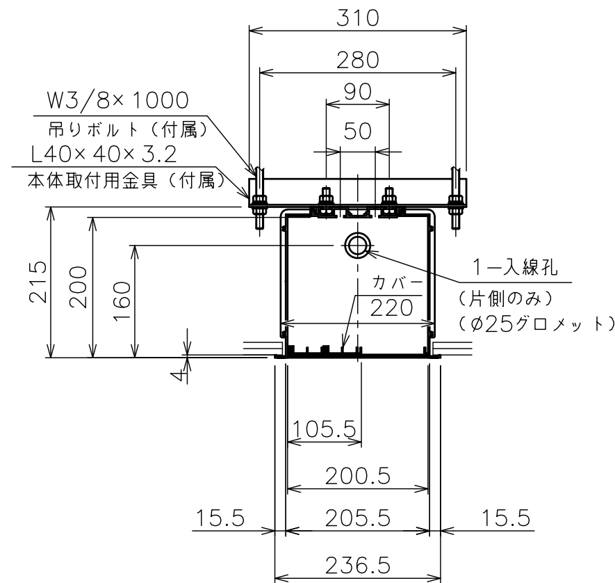
側面図詳細
