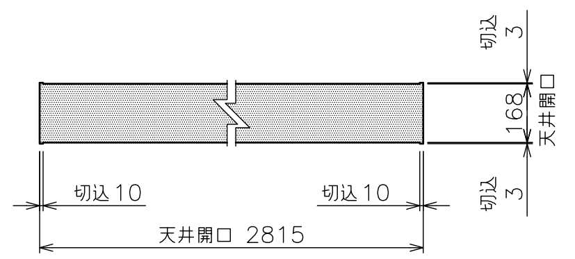
天井開口 KEYPLAN
