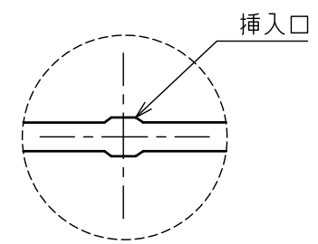
"b"部 M10ボルト挿入口拡大図
