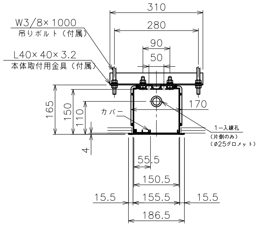
側面図詳細
