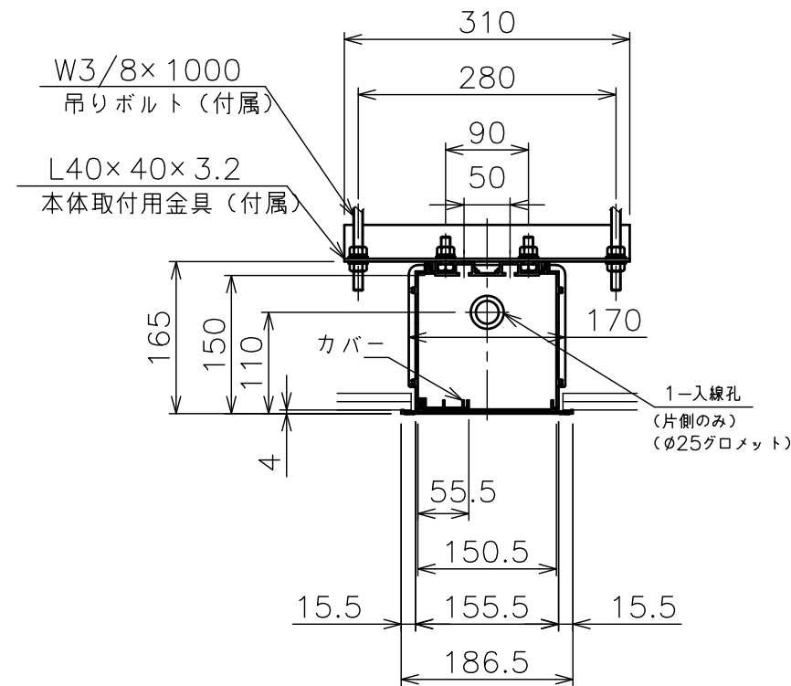
側面図詳細
