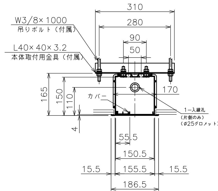
側面図詳細
