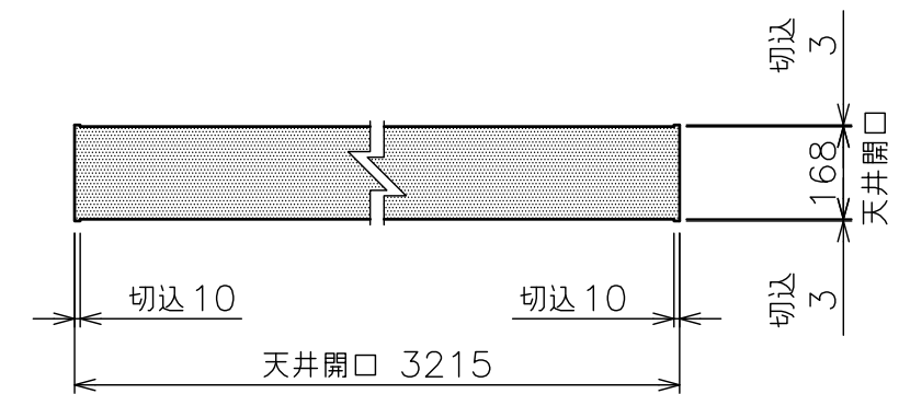
天井開口 KEYPLAN
