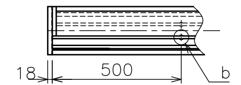
矢視 B
