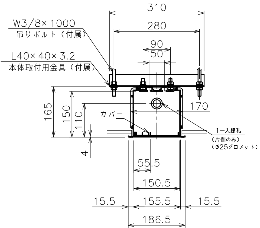
側面図詳細
