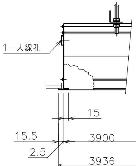
”a”部詳細
