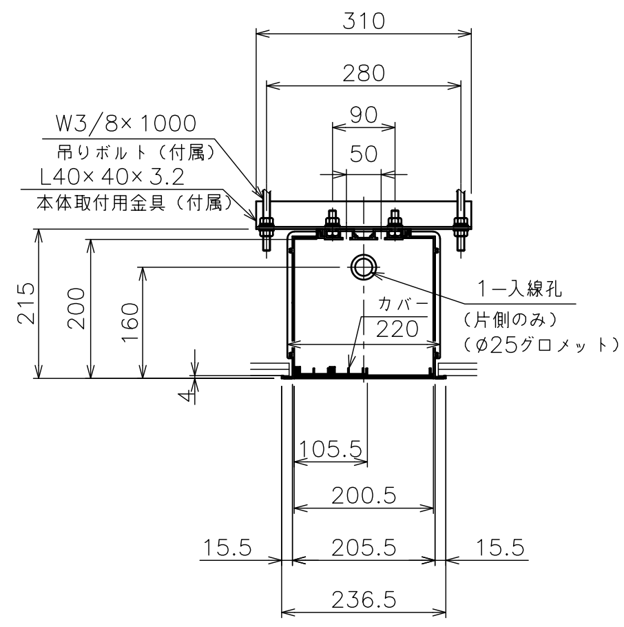
側面図詳細
