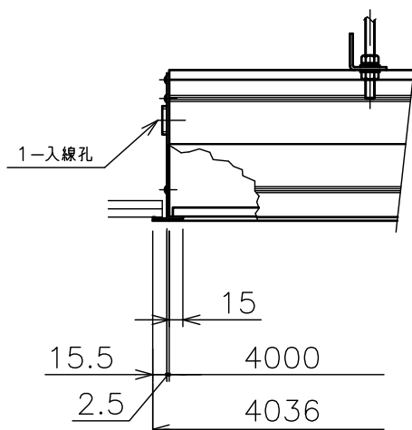
”a”部詳細
