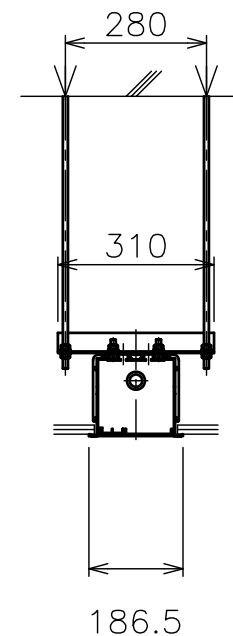
”b”部 M10ボルト挿入口拡大図
