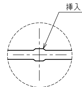
”b”部 M10ボルト挿入口拡大図
