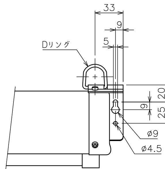
”a”部詳細
