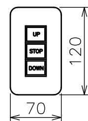
一連用埋込型スイッチ (モダンプレート：ミルクホワイト)
