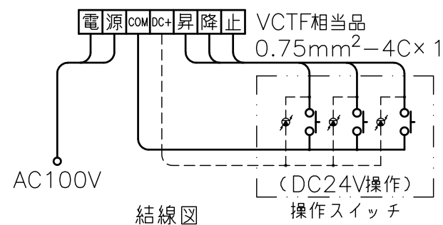
一連用埋込型スイッチ (モダンプレート：ミルクホワイト)
