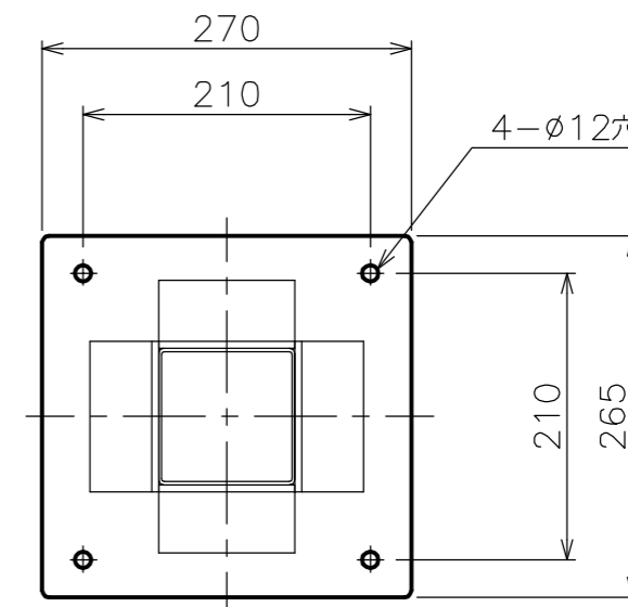
矢視 A - A <ハンドル側>
