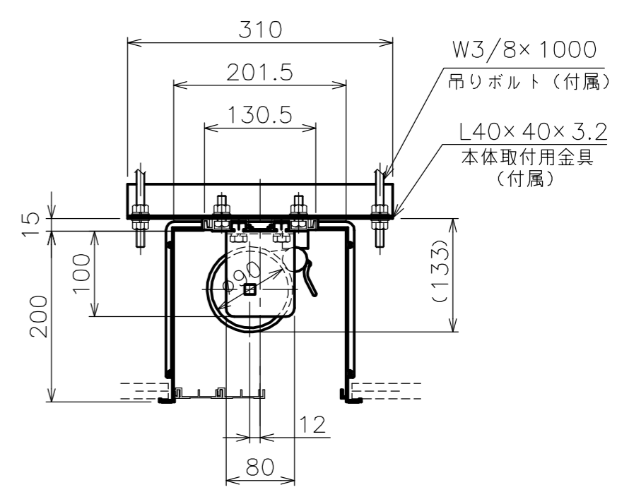
矢視 A - A
