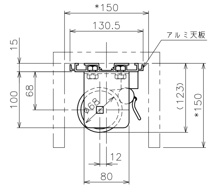
”a”部詳細
