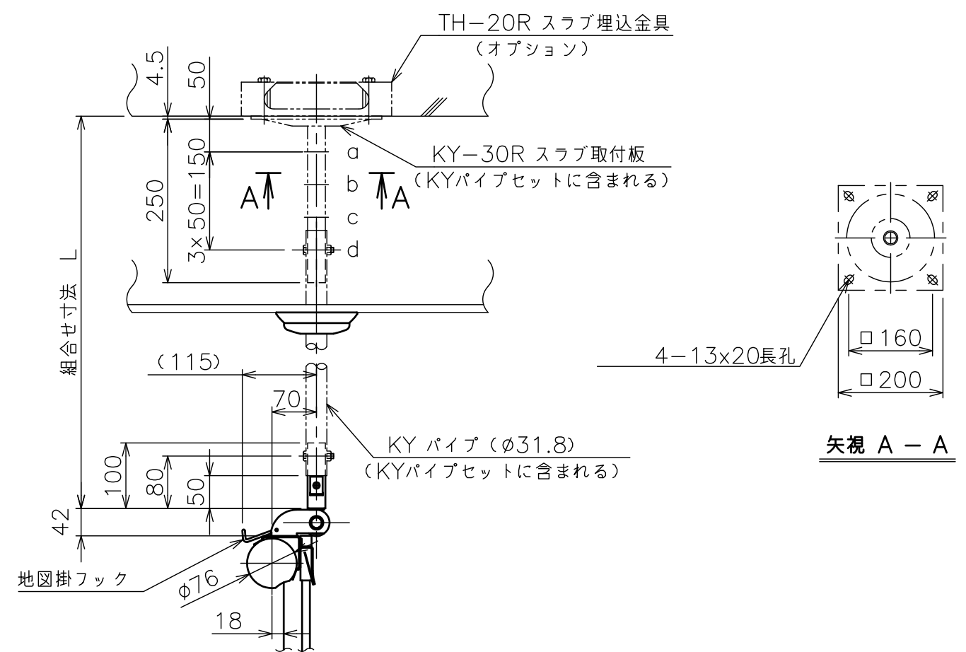
”a”部詳細
