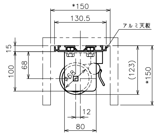
”a”部詳細
