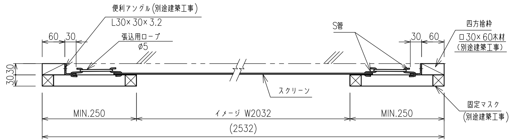
矢視 A - A (2532)
