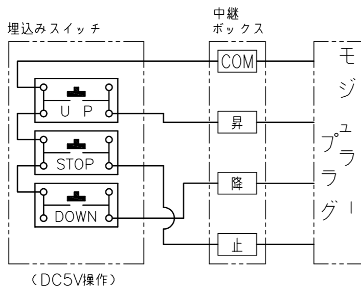
配線図
