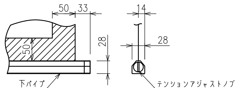
下パイプ詳細図(S=1/5)
