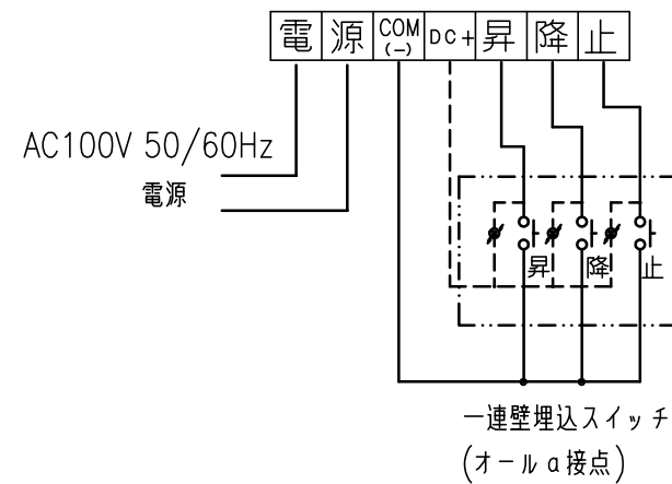
結線図
