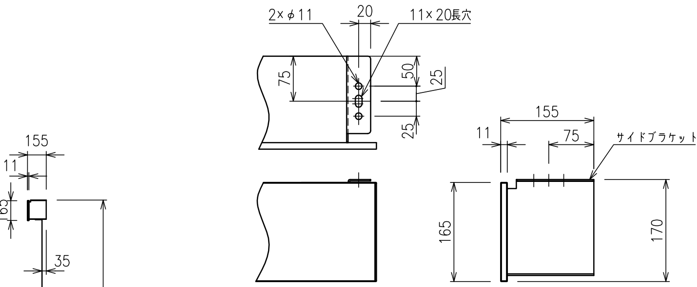
サイドブラケット詳細図(S=1/6)
