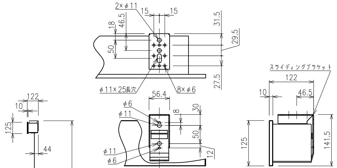
スライディングブラケット詳細図 (S=1/5)
