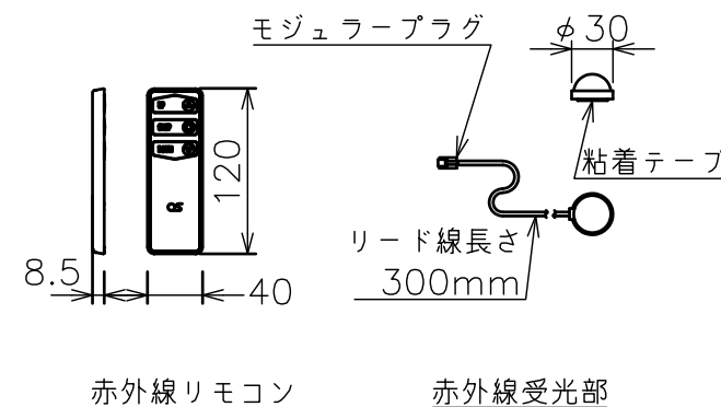
モジュラーおよびリモコン (S=1/5)
